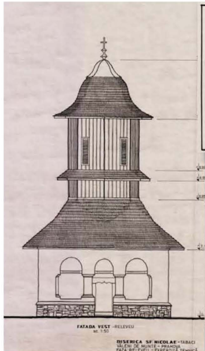
Biserica Sf. Nicolae 2006. Fațada Vest
