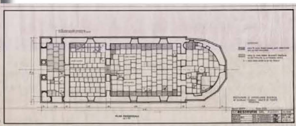
Biserica Sf. Nicolae 2006. Plan pardoseală
